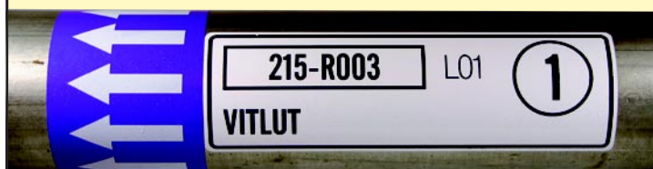
Exempel på märkning med piltejp och dekal med egen utformning. (StoraEnso Skoghalls standard: Flödesriktning, rörnummer, SSG-kod, objektgrupp och klartext anges.)
